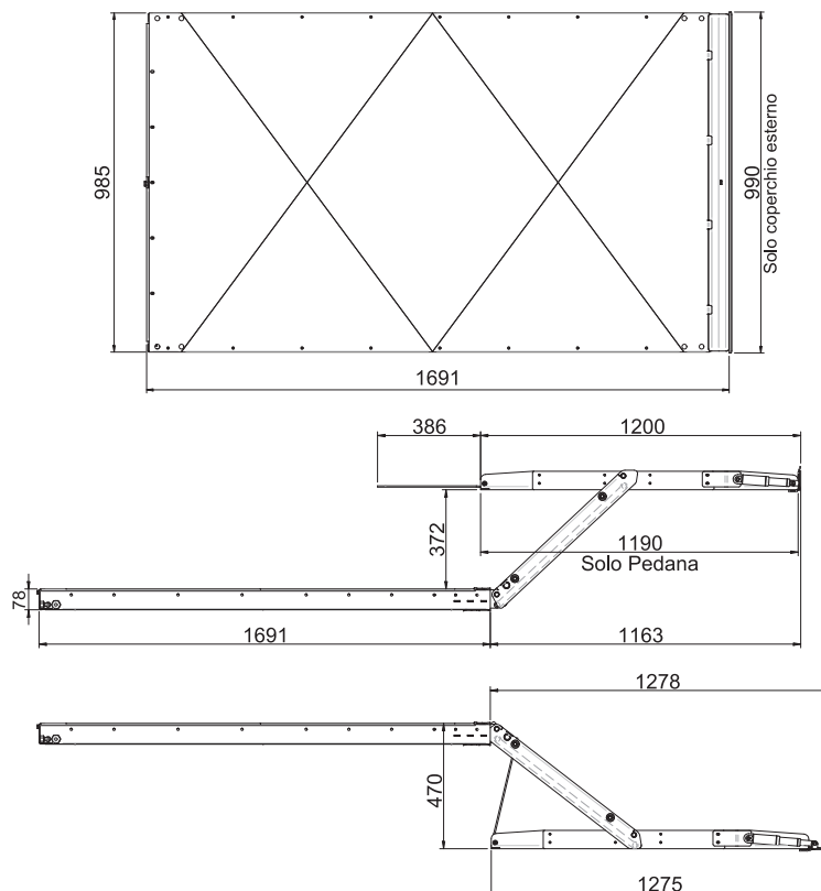
DIMENSIONS/INGOMBRI EP 300
